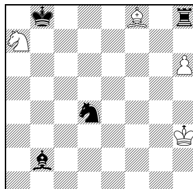
30 biely remizuje? 4+4
