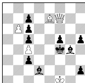
29 biely remizuje 5+10
