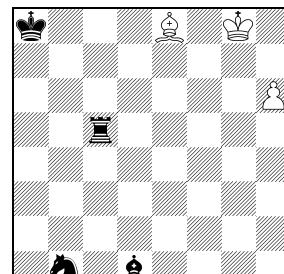
33 biely remizuje 3+4
