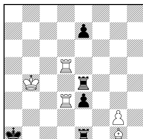
27 biely vyhrá 5+5
