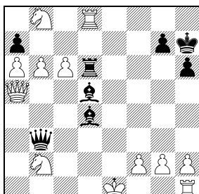
26 biely vyhrá 12+8
