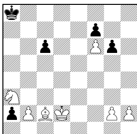
28 biely vyhrá 7+5
