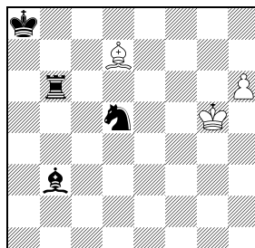
32 biely remizuje 3+4
